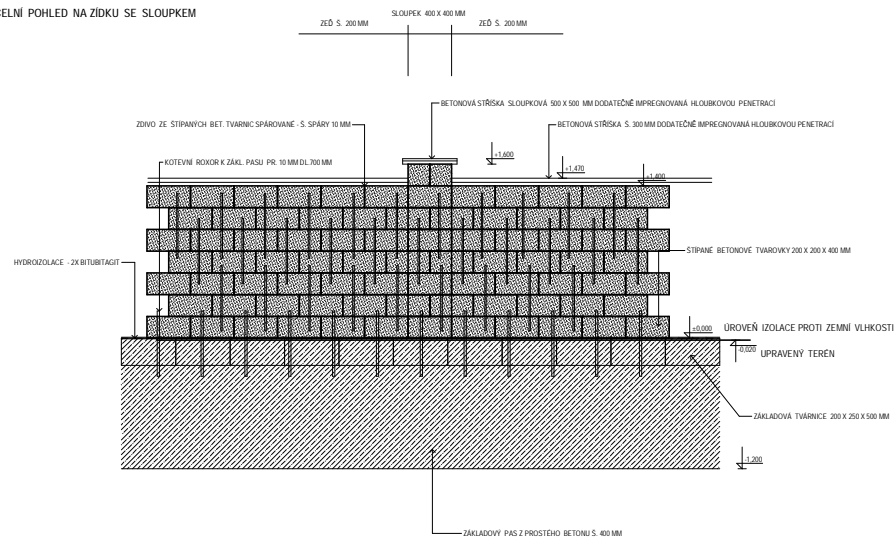
ČELNÍ POHLED NA ZIDKU SE SLOUPKEM
