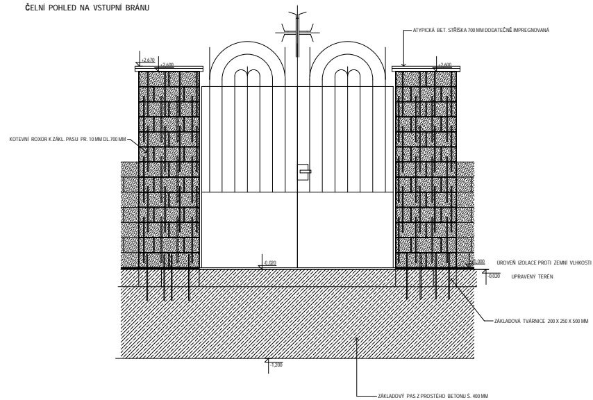
ČELNÍ POHLED NA VSTUPNÍ BRÁNU
